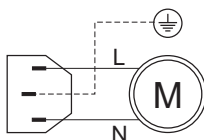
Rys. 3 Schemat podłączenia przewodu do pompy lub wentylatora
