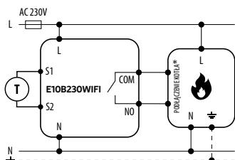
a) Schemat podłączenia do kotła gazowego
